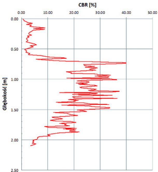
Rys. 3. Przykład prezentacji graficznej wyników CBR podłoża sondą Panda
