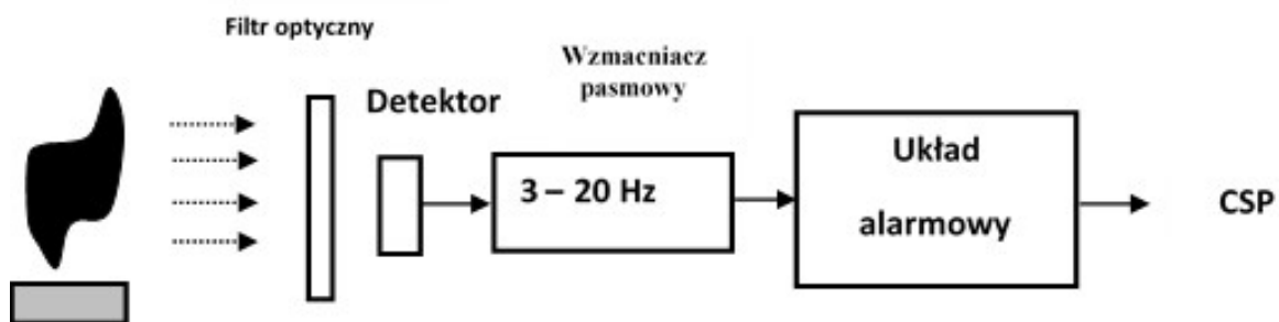
Rys. 10. Idea działania czujki płomienia działającej w zakresie podczerwieni
