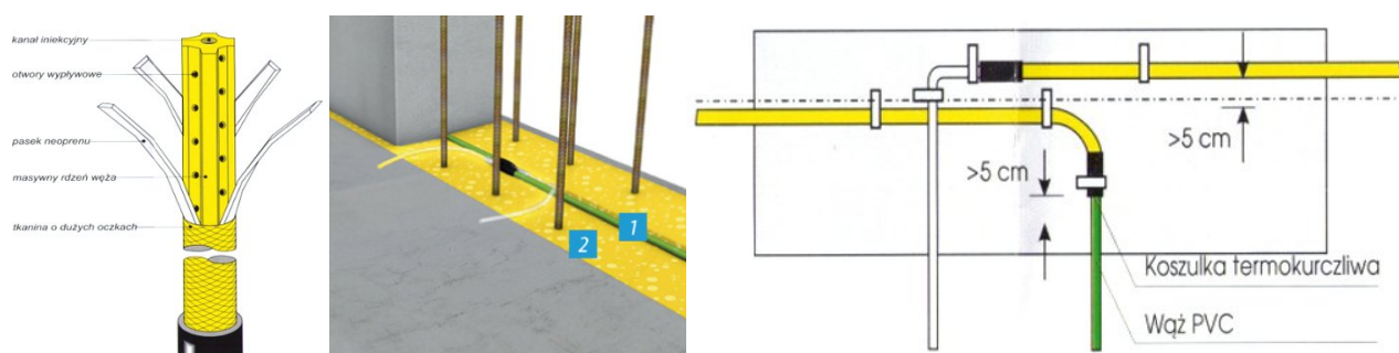
Rys. 11. Wężę do iniekcji umieszczane np. na styku płyty fundamentowej ze ścianą [14]: a) konstrukcja
