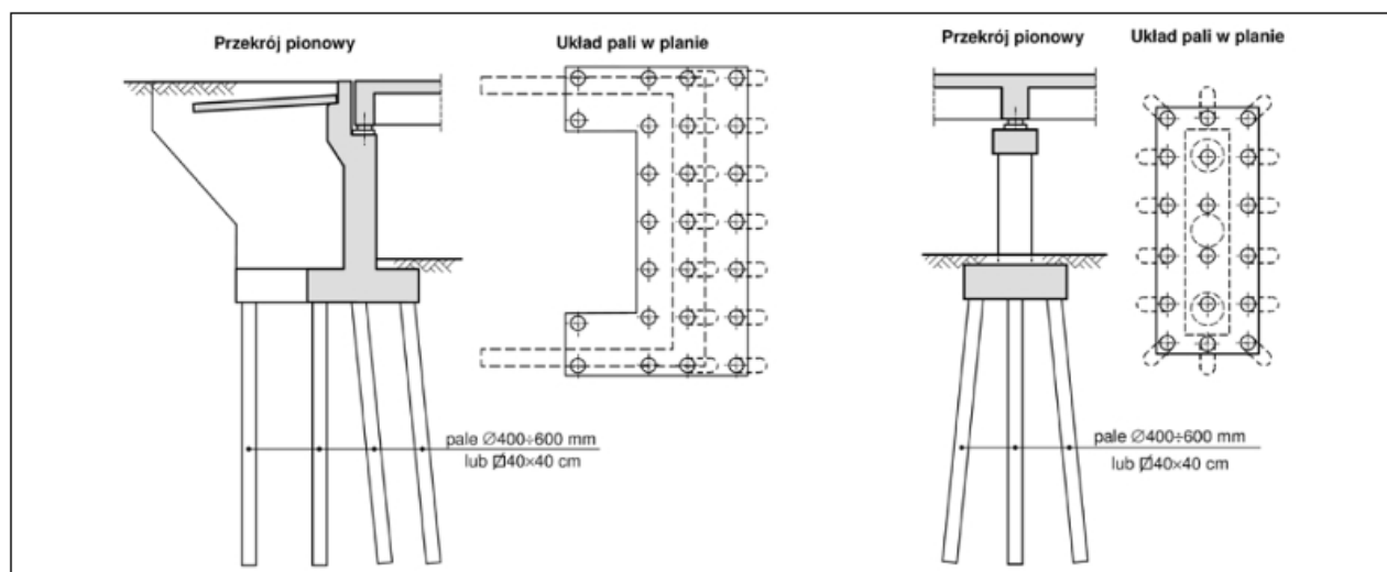
Rys. 4. Posadowienie przycółka i filara mostowego na palach wbijanych
