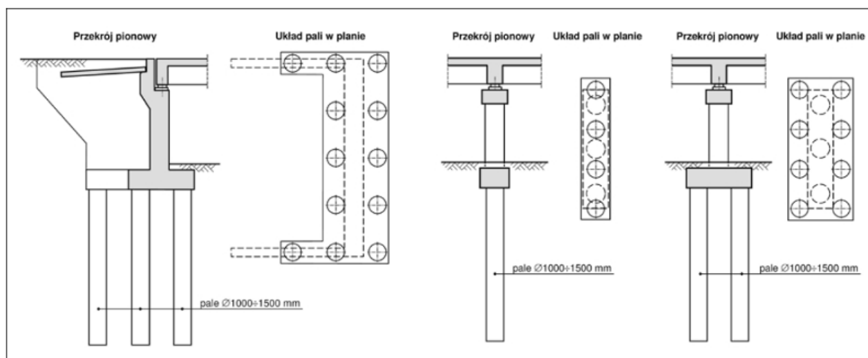
Rys. 1. Posadowienie przyczółka i filara mostowego na palach wierzonych wielkośrednicowych
