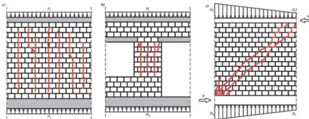
Rys. 1. Sposób zarysowania muru obciążonego w płaszczyźnie konstrukcji poddanego ścisnaniu: a) ścian nośnych, b) filarków międzyotworowych w ścianach nośnych oraz c) ścianych ścian usztywniających
