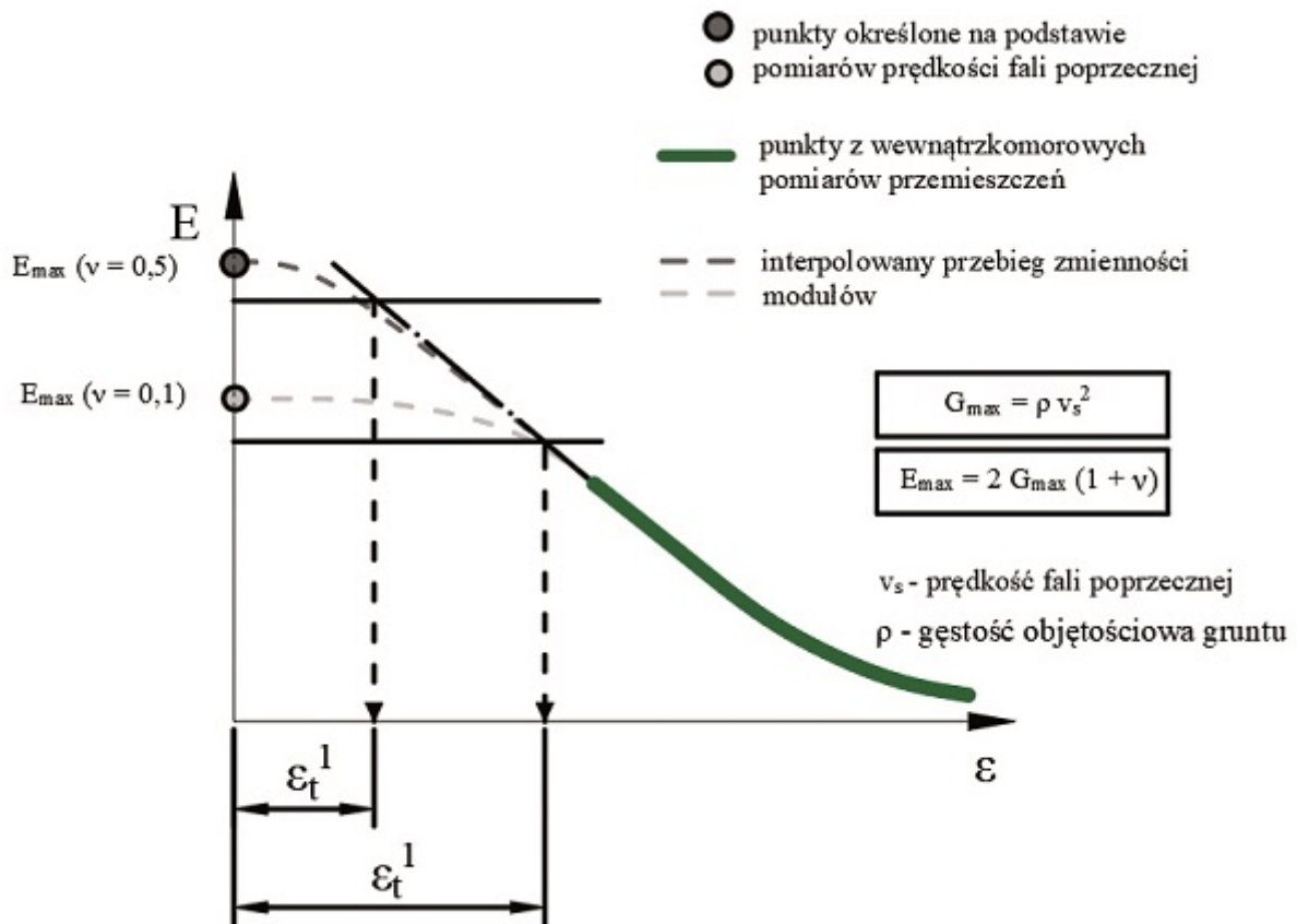
Rys. 2. Metodyka oszacowania zakresu zmienności odkształceń sprężystych [6]
